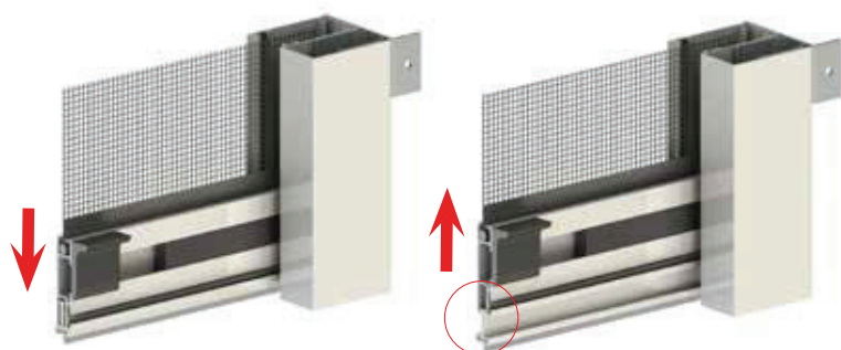
Barra maniglia con profilo portaspazzolino telescopico
