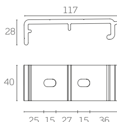
Staffa
