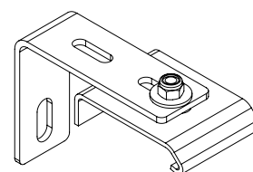
Suggerimento sul corretto montaggio (staffa a parete)
