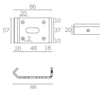
Staffe per montaggio a soffitto
