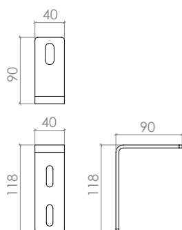
Staffa per montaggio a parete
