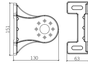
Nuova staffa attacco a parete
