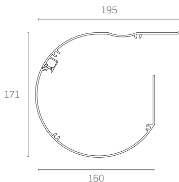
Cassonetto per sporgenze oltre a 350 cm
