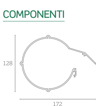
Cassonetto per sporgenze fino a 350 cm
