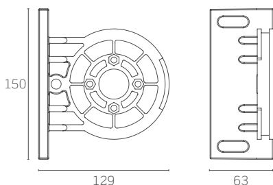
Staffa attacco a parete (Fino ad esaurim. scorte)
