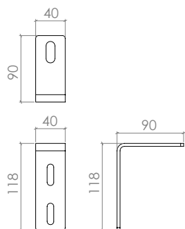
Staffa per montaggio parete
