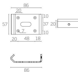
Staffe per montaggio a soffitto
