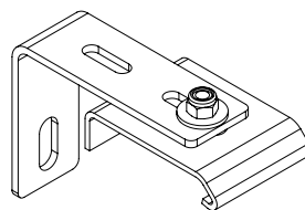
Suggerimento sul corretto montaggio (staffa a parete)
