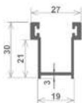
Guida cod. 30x19
