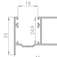
Guida con distanziale 20 cod. 35x41
