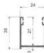
Guida cod. 30X24 (comprensivo di spazzolino maggiorato)
