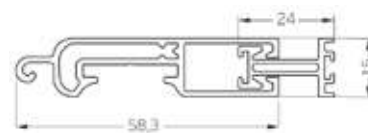
Terminale con profilo telescopico
