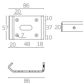
Staffe per montaggio a soffitto
