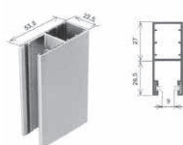
Guida in alluminio a misura per fianchi Mini
