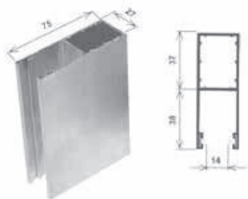
Guida in alluminio a misura per fianchi Standard
